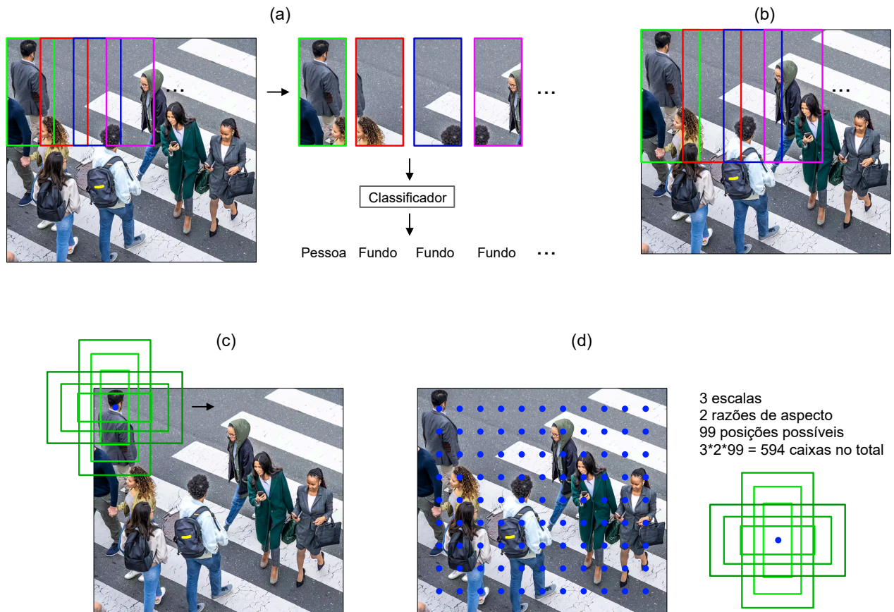
Figura 2.13: Conceitos básicos de detecção de objetos. (a) Regiões da imagem são extraídas a partir de uma janela deslizante. Cada região é classificada em uma classe distinta por um classificador. (b) O processo é repetido para uma janela de maior tamanho (escala). (c) De forma equivalente à janela deslizante, podemos considerar que pontos âncora são definidos (ponto azul), e janelas de diferentes tamanhos e razão de aspecto são associadas a cada ponto. Regiões fora da imagem possuem valor 0. (d) Uma grade de pontos âncora é definida, com k janelas associadas para cada ponto. Essas janelas são chamadas de caixas âncora .
