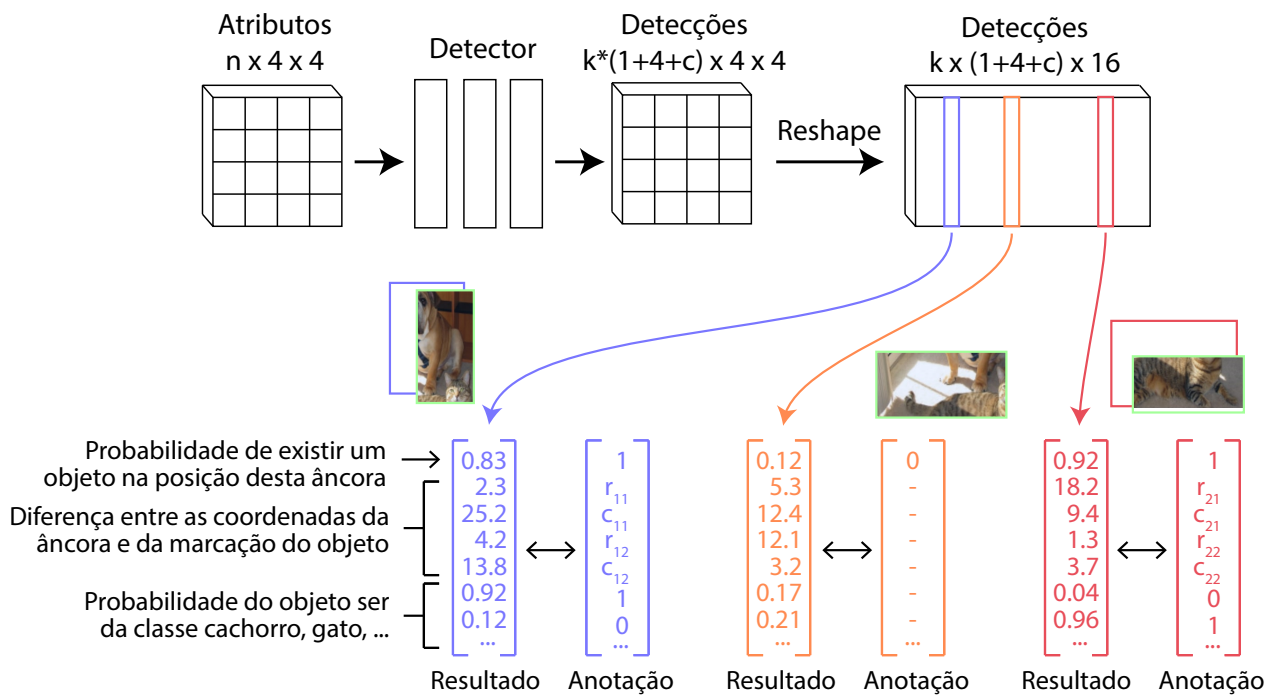
Figura 2.15: Treinamento de um modelo de detecção de objetos. Uma rede neural (detector) é aplicada nos atributos do codificador. Essa rede gera 1+4+c valores para cada posição do mapa de atributos e para cada âncora. No exemplo, o mapa de atributos possui 4 \times 4 = 16 posições e cada posição possui k caixas âncora. c é o número de classes presentes nos dados. Exemplos de valores para três âncoras são mostrados, eles correspondem às âncoras com maior intersecção com a anotação do cachorro (azul) e do gato (vermelho) e uma âncora que não possui nenhum objeto (laranja). Os resultados da rede são comparados com as anotações manuais. O primeiro valor representa a probabilidade da âncora possuir um objeto válido. Os próximos 4 valores representam o deslocamento previsto pelo detector para que a âncora represente de forma mais adequada a posição do objeto na imagem. Os c valores restantes representam as probabilidades do objeto na posição da âncora ser de cada classe. Os valores de classe são independentes, isto é, eles não somam 1. Isso é feito para que seja possível realizar uma classificação multirótulo. Os valores de probabilidade são otimizados usando a entropia cruzada, enquanto que os deslocamentos das âncoras são otimizados utilizando diferenças quadráticas. Quando uma âncora não possui objetos válidos (mostrada em laranja), os valores de deslocamento e de classe são ignorados.
