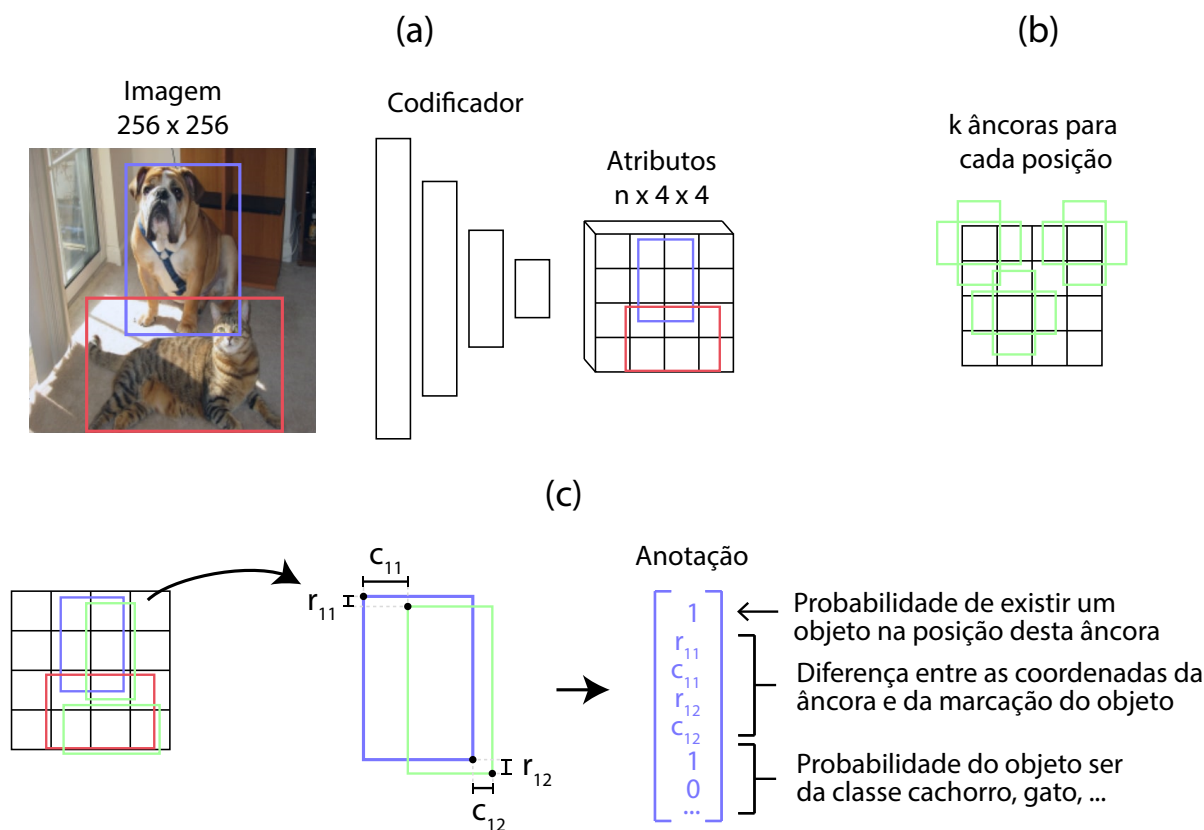
Figura 2.14: Anotação de um dataset para detecção de objetos. (a) Uma imagem passa por um codificador (ex: ResNet), que gera um mapa de n atributos de tamanho s \times s . No exemplo, o mapa possui tamanho 4 \times 4 . As posições dos objetos na imagem, anotadas manualmente, possuem uma posição equivalente no mapa de atributos. (b) Caixas âncoras são definidas para cada posição possível do mapa de atributos. Em geral, são definidos 3 formatos de caixa (quadrada, retangular vertical e retangular horizontal) e 3 tamanhos distintos (pequena, média e grande), totalizando k=9 caixas. A figura mostra duas caixas em três posições distintas para ilustrar o conceito. (c) A diferença entre a posição das âncoras e das anotações é calculada e armazenada. Alguns métodos consideram apenas a âncora com maior intersecção com a anotação, outros consideram todas as âncoras com intersecção maior que um valor limiar predeterminado. Para cada âncora, é gerada uma anotação possuindo 1+4+c valores. O primeiro valor indica a presença ou não de um objeto na âncora. Os próximos 4 valores indicam o deslocamento que deve ser aplicado na âncora para que ela represente de forma mais adequada a posição do objeto na imagem. O c valores seguintes indicam a presença de cada classe do dataset na âncora. Caso a âncora não possua um objeto anotado, os 4+c valores não são calculados. Note que para calcular essa diferença não é necessário aplicar o codificador na imagem. Esses valores são calculados antes do início do treinamento da rede.
